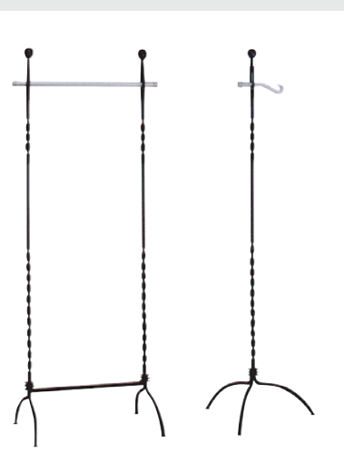
ZZ 139 W:700 D:460 H:1750 クラフトガラス スチール/CrメッキH.L クラフト風仕上 ZZ 140+KP 2265 W:560 D:490 H:1750 クラフトガラス スチール/CrメッキH.L クラフト風仕上
